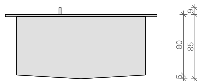
Ansicht B
